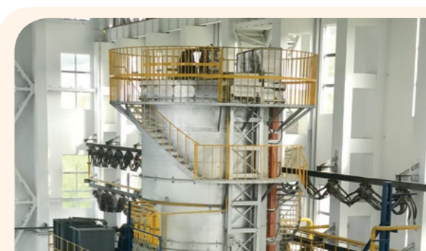
大型保护气氛联合井式炉组
